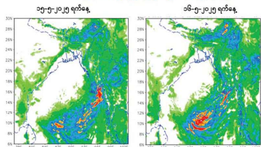
၁၅-၅-၂၀၂၅ ရက်နေ့မှ ၁၆-၅-၂၀၂၅ ရက်နေ့အတွင်း မိုးလေဝသ သင်္ချာပုံစံပြုမော်ဒယ်မှ ခန့်မှန်းထားသည့် မိုးရွာသွန်းမှုအခြေအနေ ခန့်မှန်းချက်ပြပုံ
